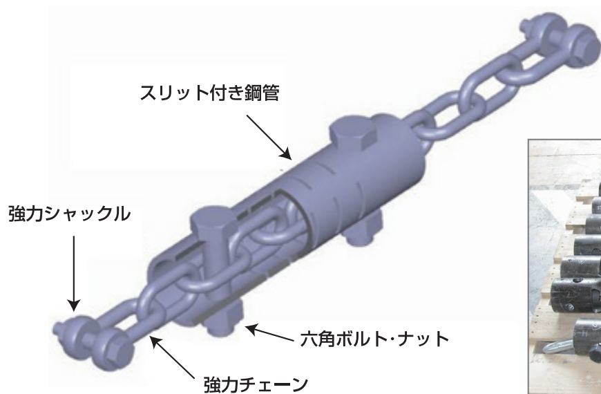
エネルギー吸収型チェーン式落橋防止装置の設置イメージ
